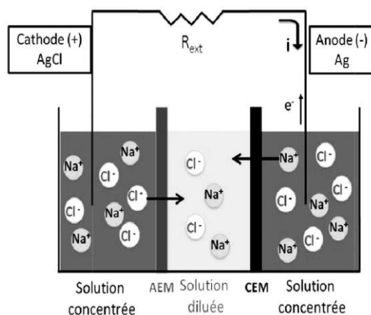
Figure 6 - Schéma d'une pile à électrodialyse inverse
