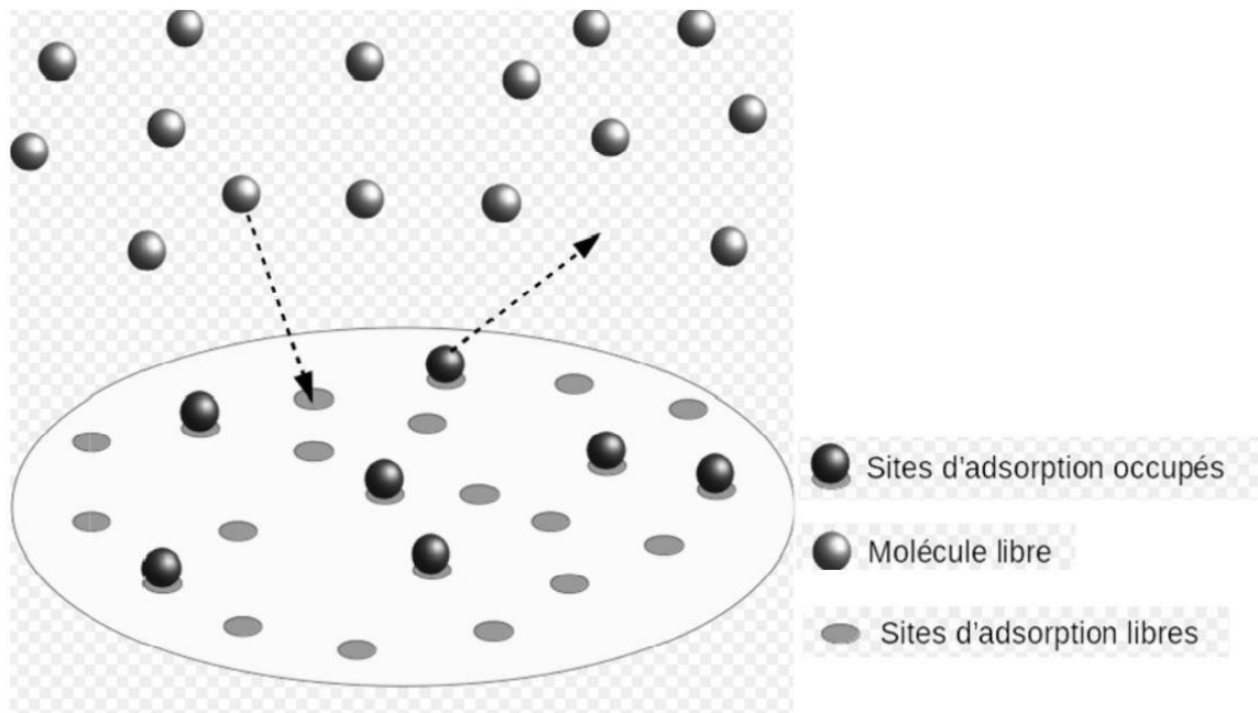
Figure 3 - Schématisation du phénomène d'adsorption sur une surface
