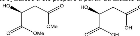
Figure 8 - Représentation topologique respective du malate de diméthyle et de l'acide malique
