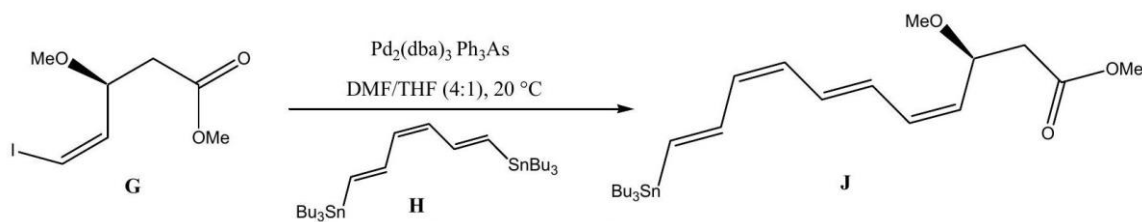
Schéma 2 - Couplage de Stille
