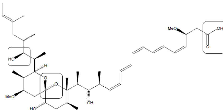
Figure 7 - Représentation topologique du (-)-spirangien
