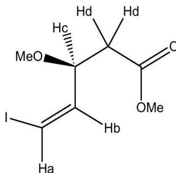
Figure 9 – Structure du composé G
