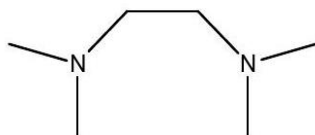
Figure 10 – Représentation topologique du TMEDA
