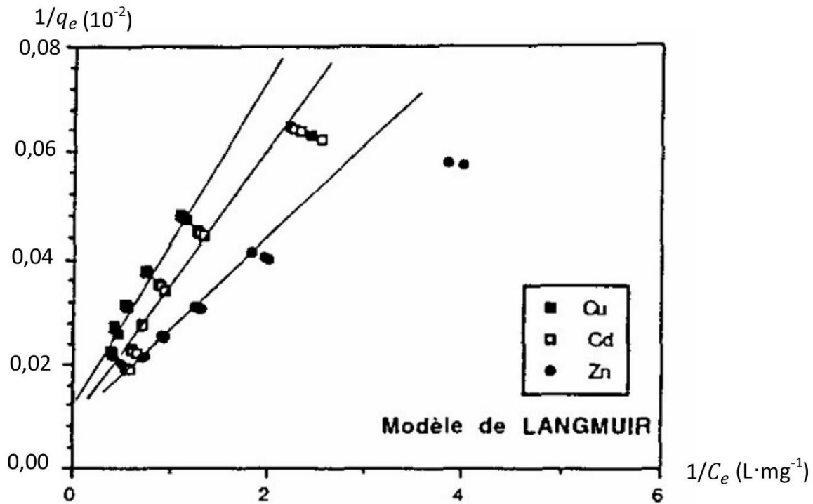
Figure 4 - Représentation linéaire des isothermes d'adsorption
