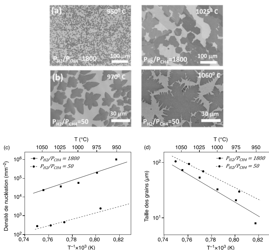
(a) Images MEB (microscopie électronique à balayage) de croissances hexagonales à différentes températures pour \frac{P_{H_2}}{P_{CH_4}} = 1800 . (b) Images MEB de croissances dendritiques à différentes températures pour \frac{P_{H_2}}{P_{CH_4}} = 50 . Diagrammes d'Arrhénius pour (c) la densité de nucléation et (d) la taille des grains.
