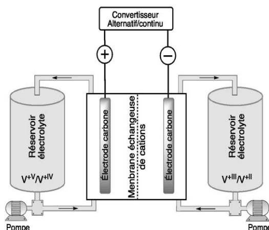
Figure 2. Schéma de principe d'une batterie à flux rédox.
