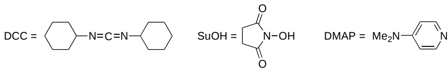
Schéma 7. Synthèse du complexe de ruthénium 11 .
